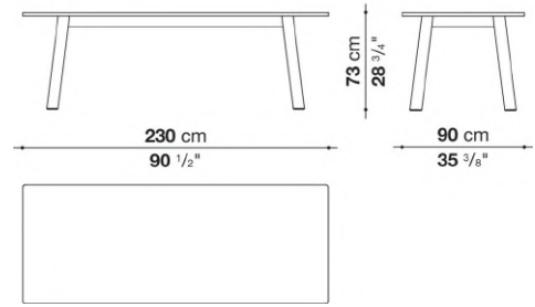
TBU230M
