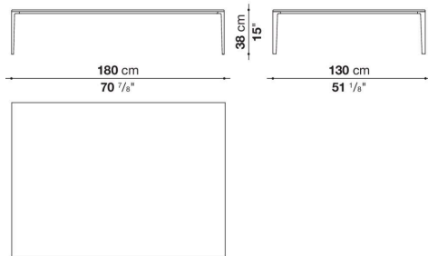
LXT180M
